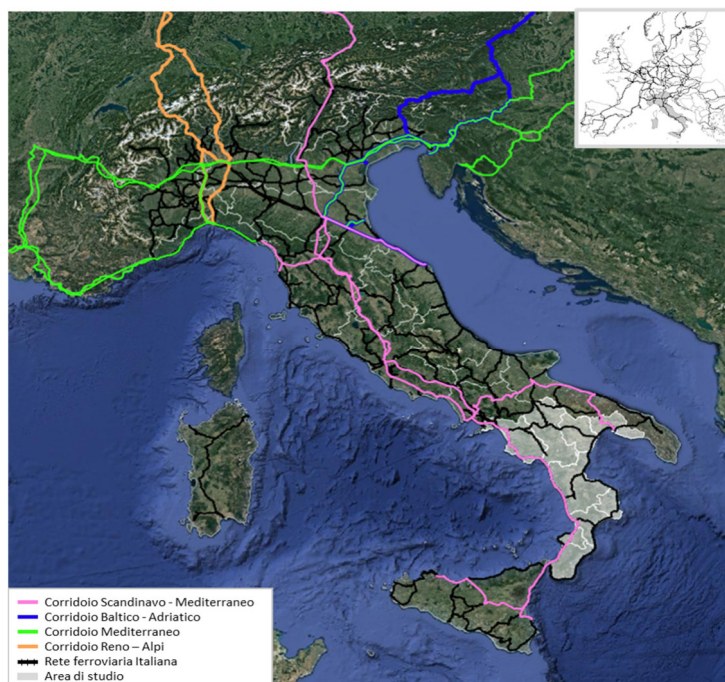
Rete dei corridoi TEN-T sul territorio italiano.
