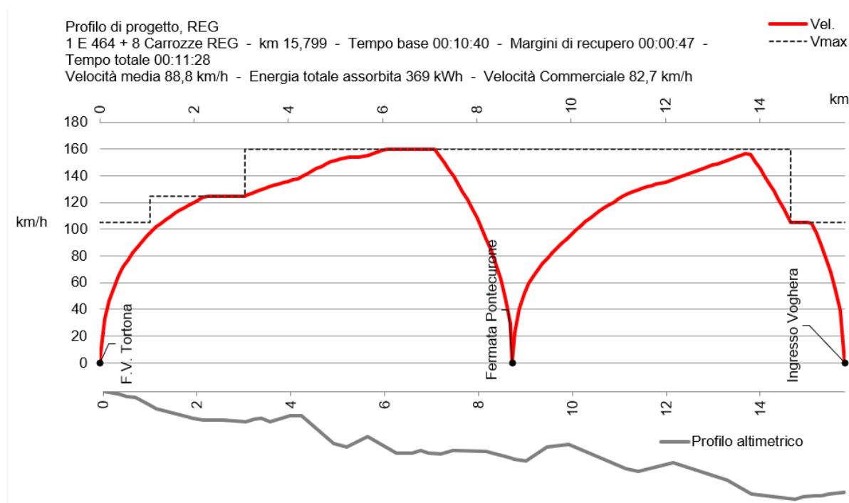
Figura 11 – Simulazione di marcia, servizio Regionale, scenario di progetto
