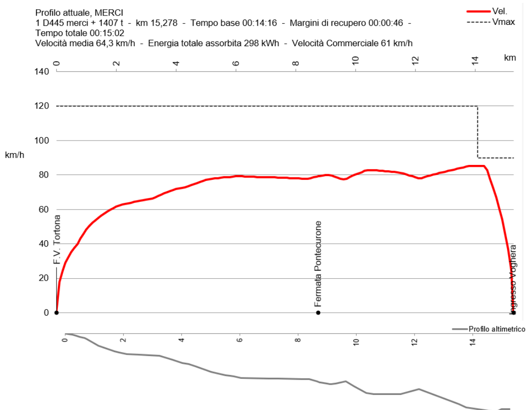
Figura 10 – Simulazione di marcia, servizio Merci, scenario attuale
