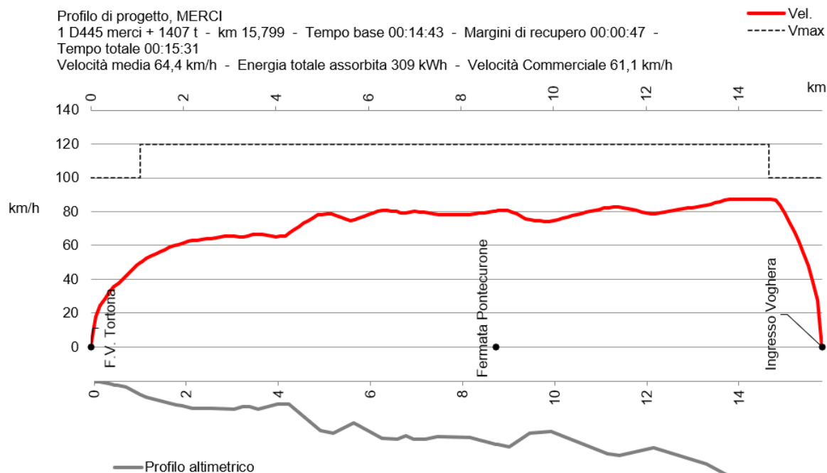
Figura 14 – Simulazione di marcia, servizio Merci, scenario di progetto
