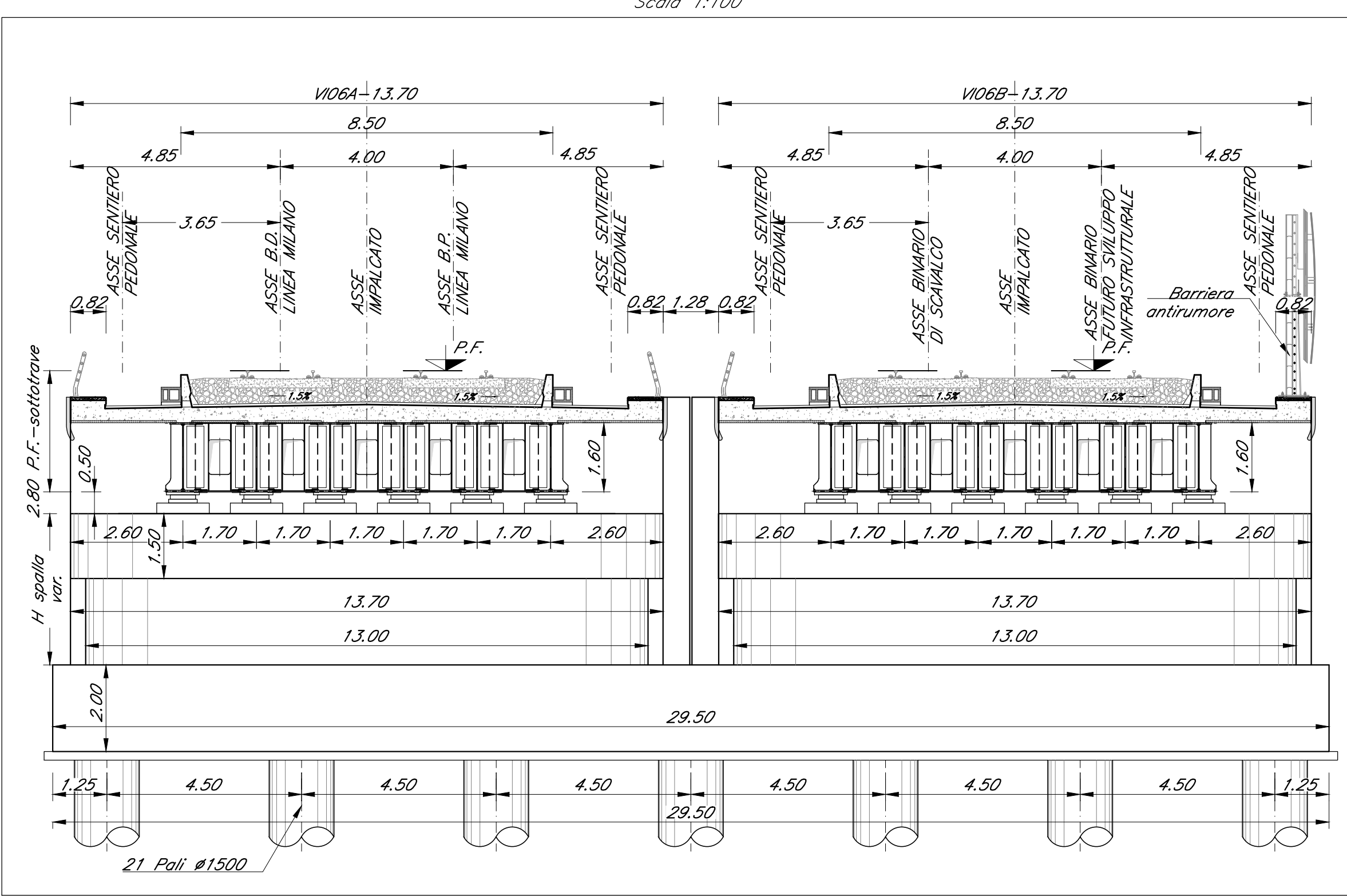
SEZIONE TRASVERSALE TIPO
