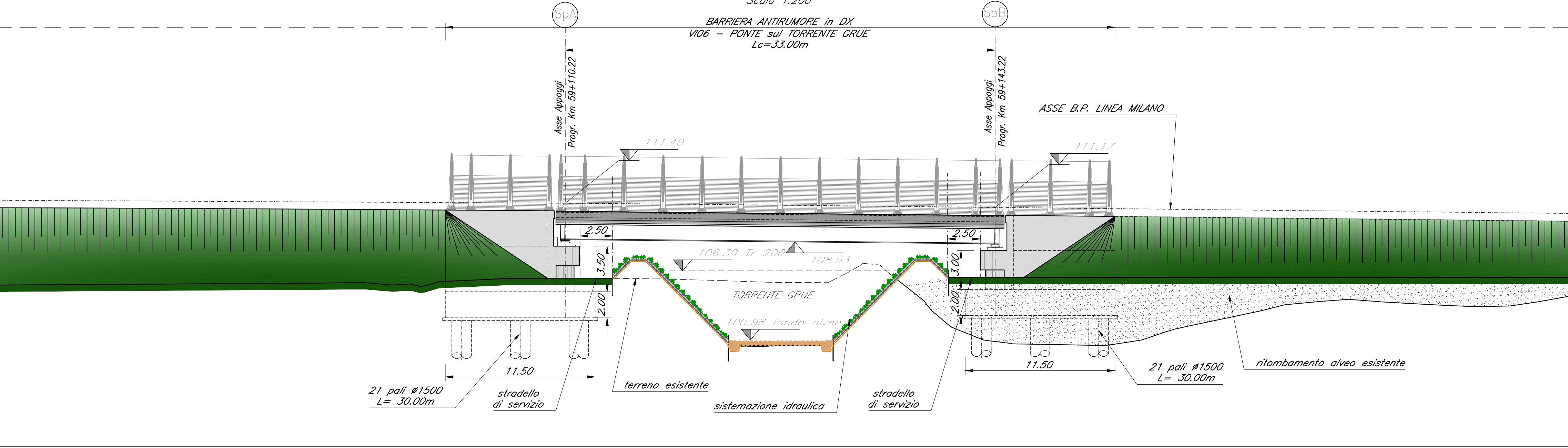
PROSPETTO/SEZIONE LONGITUDINALE
