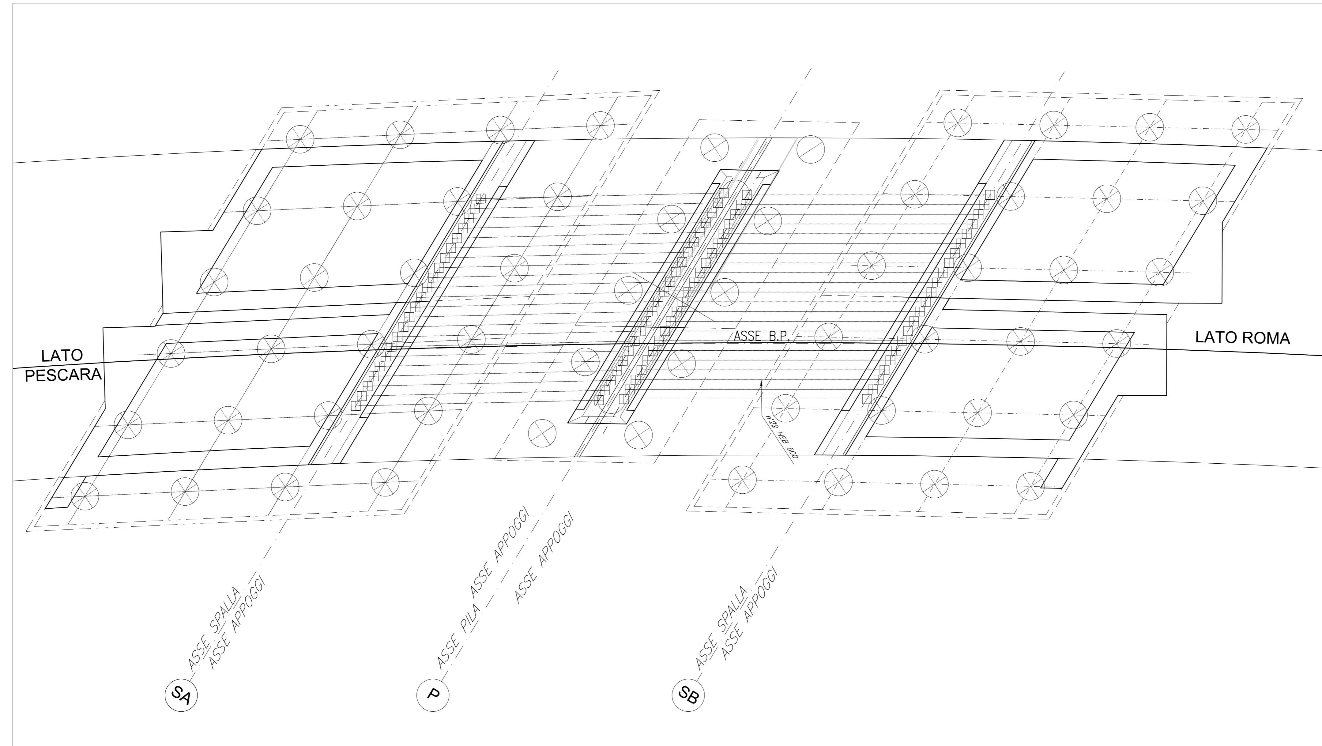
PLANIMETRIA IMPALCATO Scala 1:100
